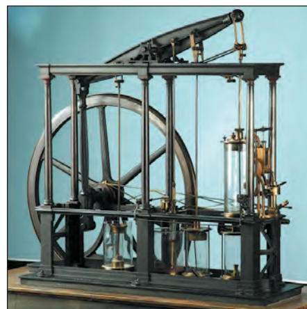
Парова машина, зроблена за проектом Дж. Ватта
